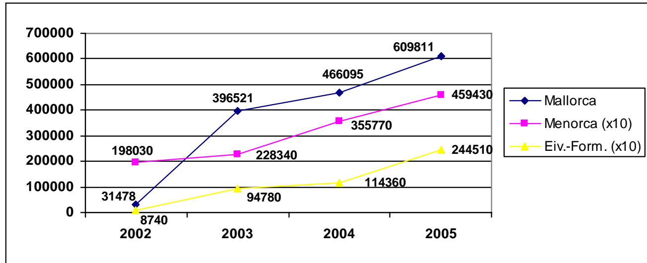
Gràfic A I-18 Evolució de l'energia d'origen fotovoltaic
