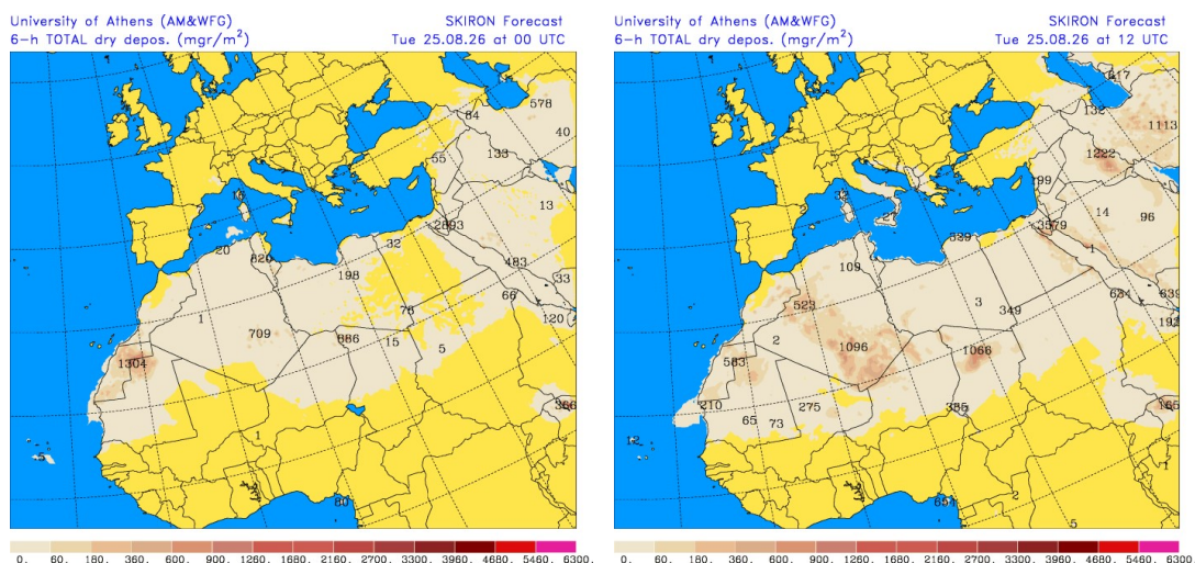
Dépósito seco de polvo ( \text{mg}/\text{m}^2 ) predicho por el modelo SKIRON para el día 25 de agosto de 2026 a las 00 UTC (izquierda) y a las 12 UTC (derecha). © Universidad de Atenas.
