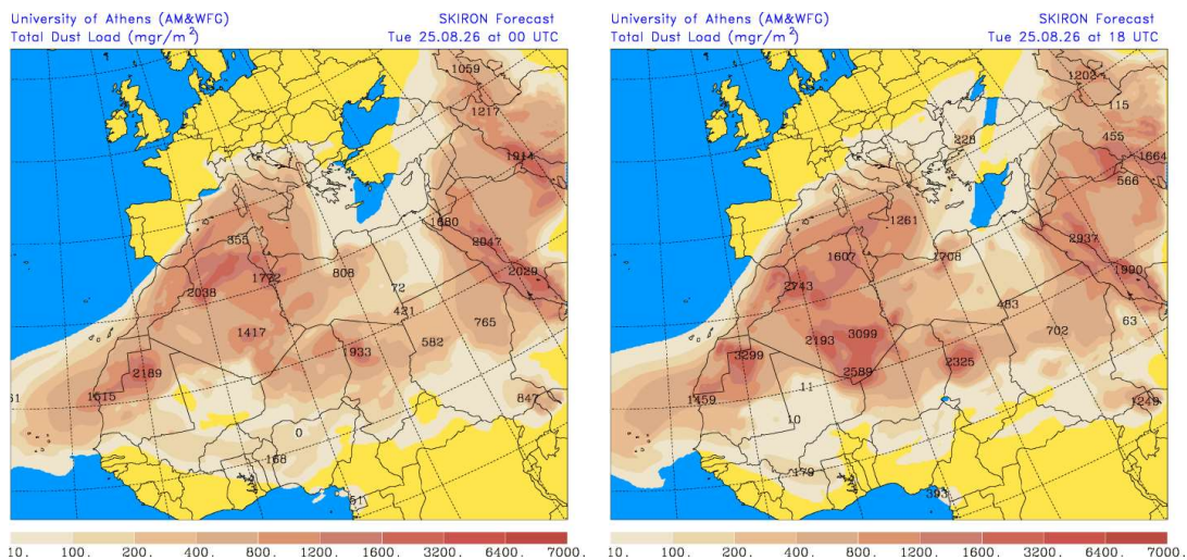
Carga total de polvo ( \text{mgr}/\text{m}^2 ) predicha por el modelo Skiron para el día 25 de agosto de 2026 a las 00 (izquierda) y a las 18 UTC (derecha). © Universidad de Atenas.
