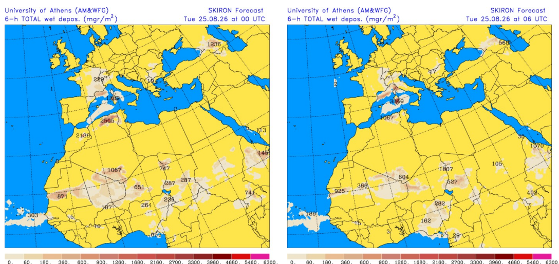
Dépósito húmedo de polvo ( \text{mg}/\text{m}^2 ) predicho por el modelo SKIRON para el día 25 de agosto de 2026 a las 00 UTC (izquierda) y a las 06 UTC (derecha). © Universidad de Atenas.
