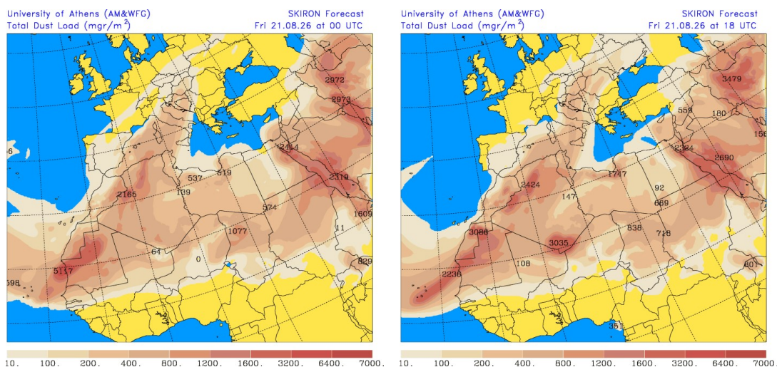
Carga total de polvo ( \text{mgr}/\text{m}^2 ) predicha por el modelo Skiron para el día 21 de agosto de 2026 a las 00 (izquierda) y a las 18 UTC (derecha). © Universidad de Atenas.
