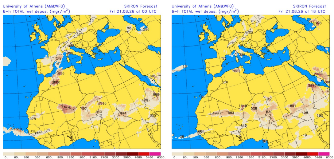
Depósito húmedo de polvo ( \text{mg}/\text{m}^2 ) predicho por el modelo SKIRON para el día 21 de agosto de 2026 a las 00 UTC (izquierda) y a las 18 UTC (derecha). © Universidad de Atenas.
