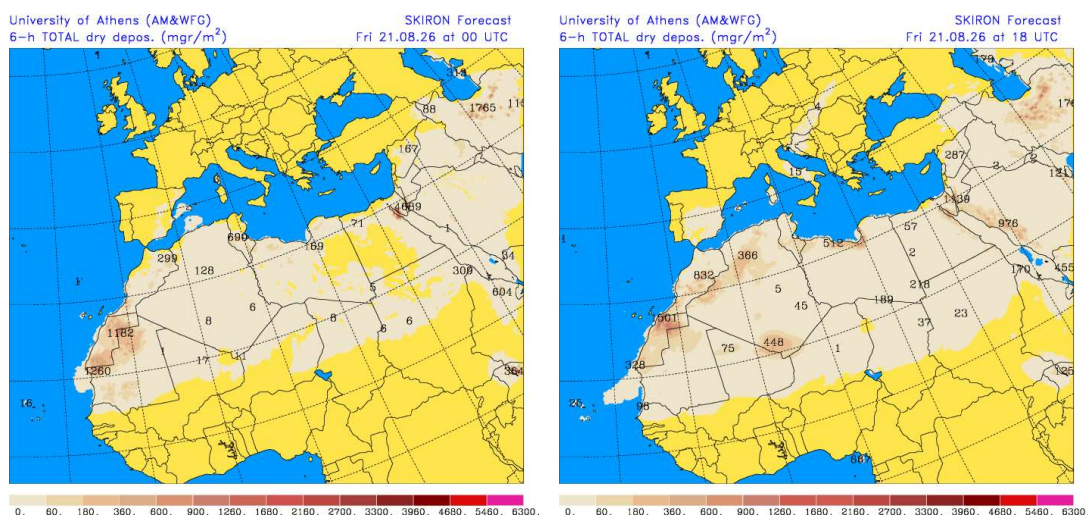
Depósito seco de polvo ( \text{mg}/\text{m}^2 ) predicho por el modelo SKIRON para el día 21 de agosto de 2026 a las 00 UTC (izquierda) y a las 18 UTC (derecha). © Universidad de Atenas.
