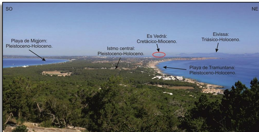
Panorámica de Formentera vista desde Es Mirador, con los principales rasgos geológicos observables en el paisaje
