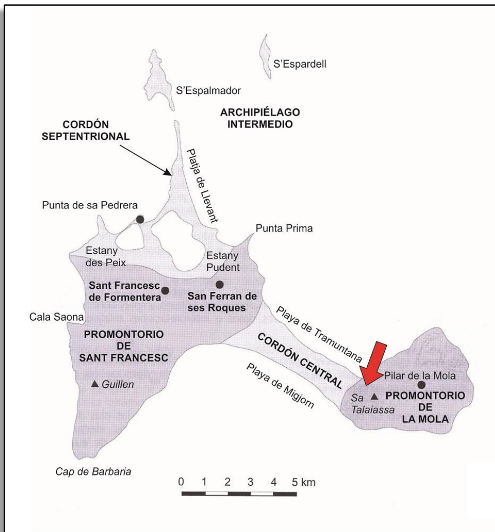
Estructuración de Formentera. Modificado de IGME, 2009.
