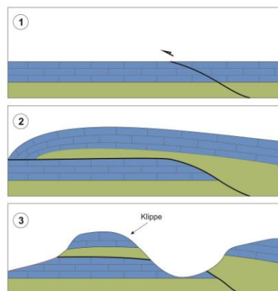
Esquema de la gènesi d'un klippe tectònic
