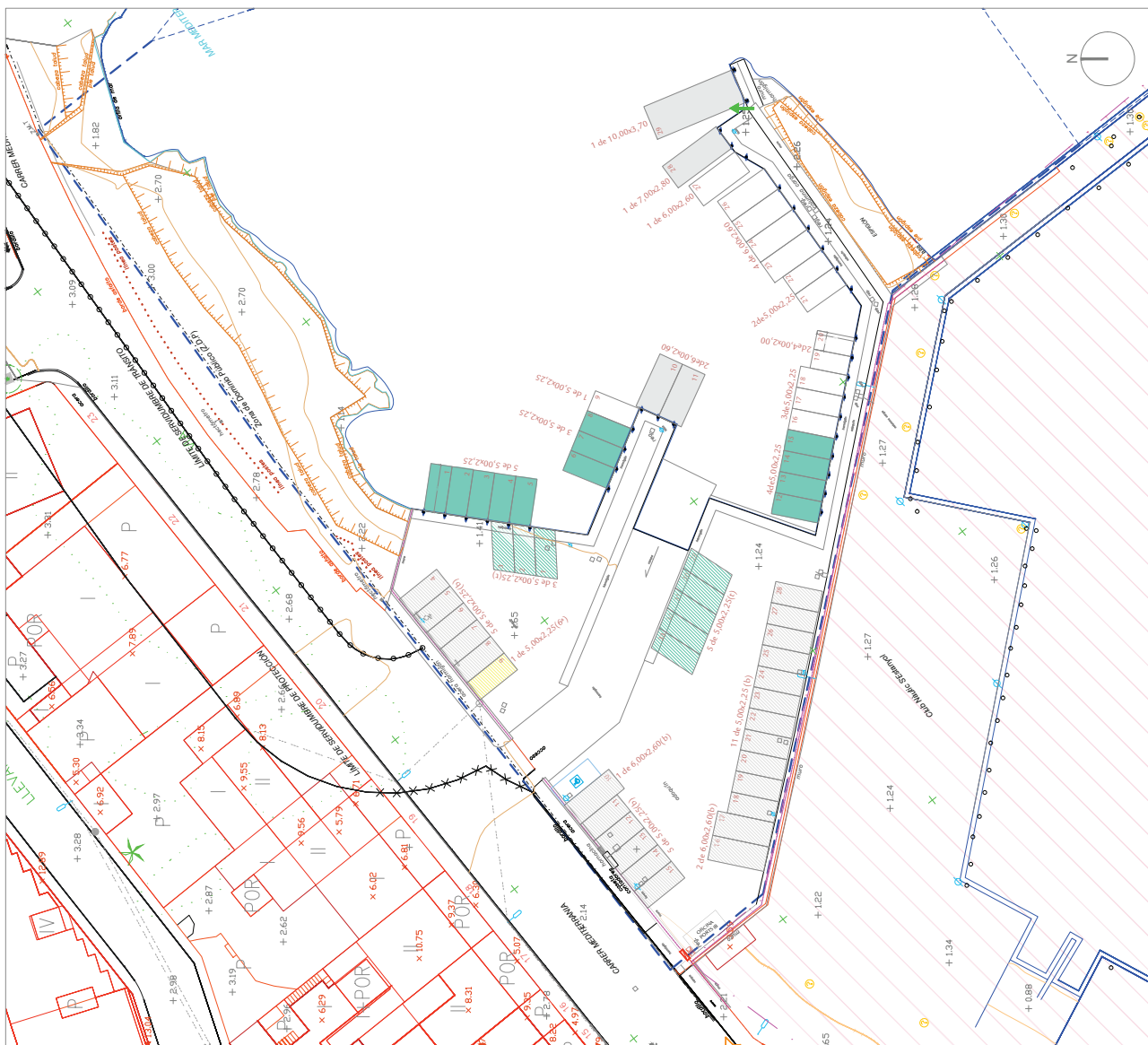
PLANTA GENERAL DEL PUERTO DE S'ESTANYOL E:1/2500
