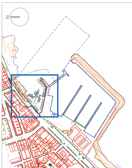
PLANTA GENERAL DEL PUERTO DE S'ESTANYOL E:1/2500
