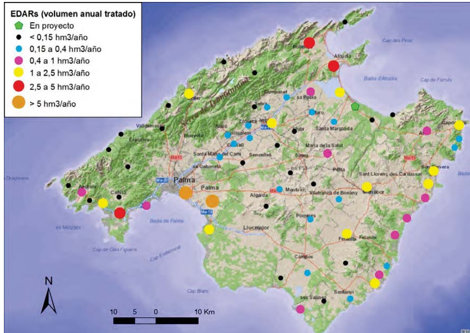
Figura 12 EDAR existentes y en proyecto en Mallorca
