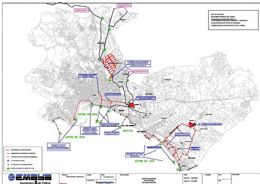
Figura 13 Obras previstas en el Plan Director de saneamiento de la Bahía de Palma
