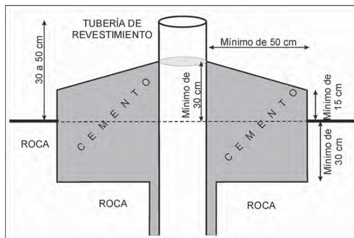
Figura 2.- Cierre o boca de la captación.
