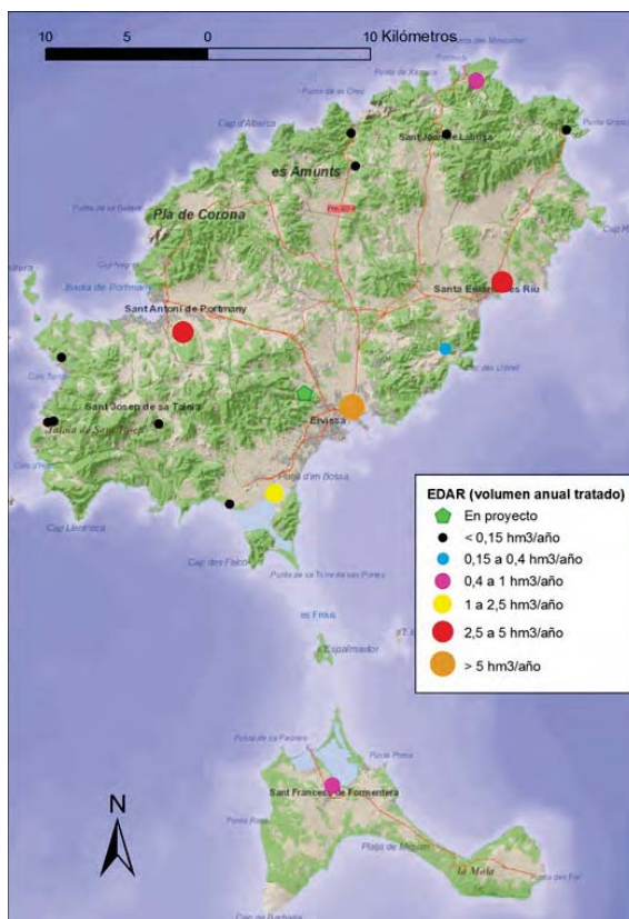
Figura 11 EDAR existentes y en proyecto en Pitiüses.
