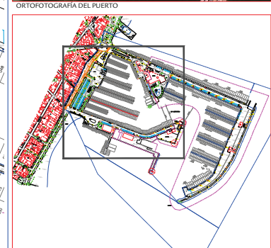
PLANTA GENERAL PUERTO DE POLLENÇA s/n
