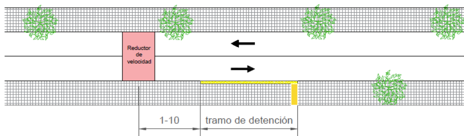
Figura 6.15: Parada urbana sin apartadero y con resalto
