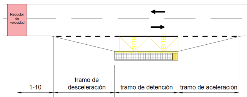
Figura 6.17: Parada interurbana con apartadero y con resalto
