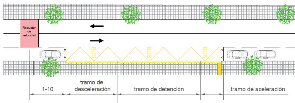
Figura 6.16: Parada urbana con apartadero y con resalto
