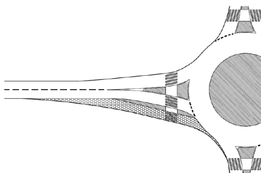
Figura 8.16: Parada interurbana con apartadero y carril propio agregado antes de rotonda (Fig. 3.5-D de la Guía de nudos viarios)
