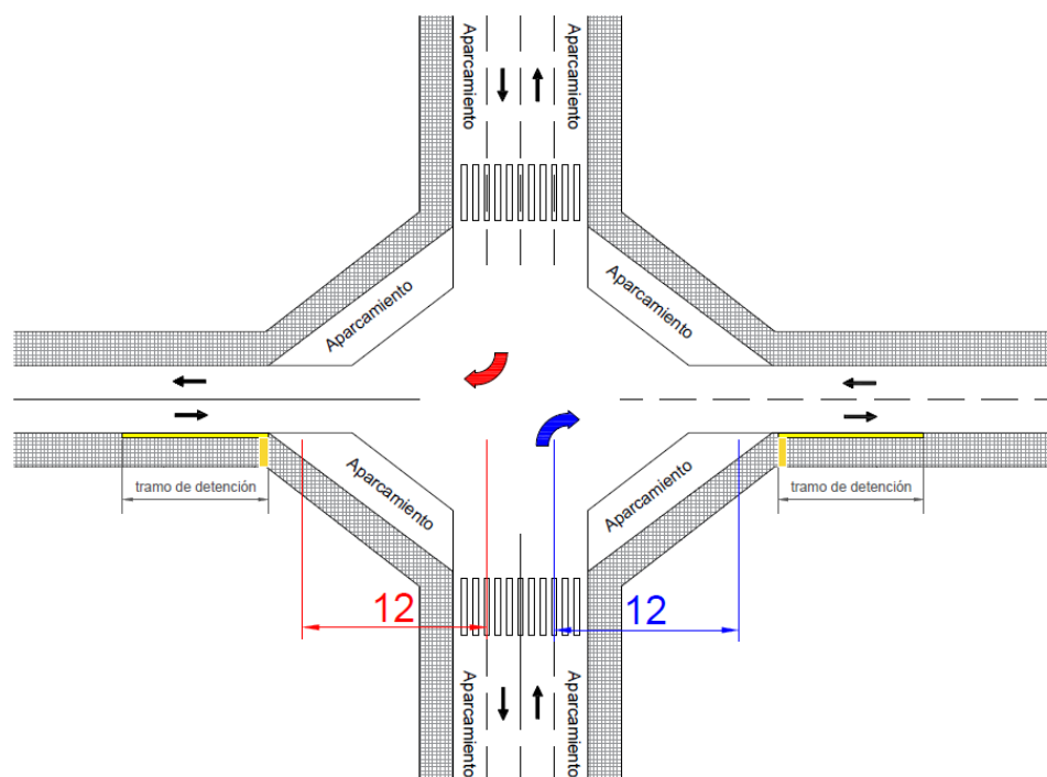
Figura 7.14: Distancias recomendadas respecto a intersección con chafalán de grandes dimensiones
