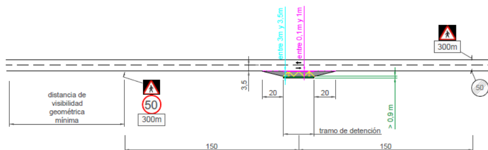
Figura 8.10: Distancias de señalización a parada interurbana con apartadero en tramo de velocidad 50 km/h
