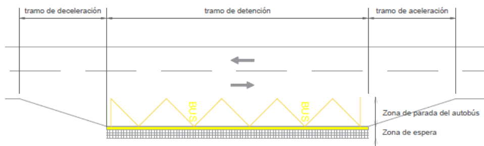
Figura 4.2: Elementos parada de autobús
