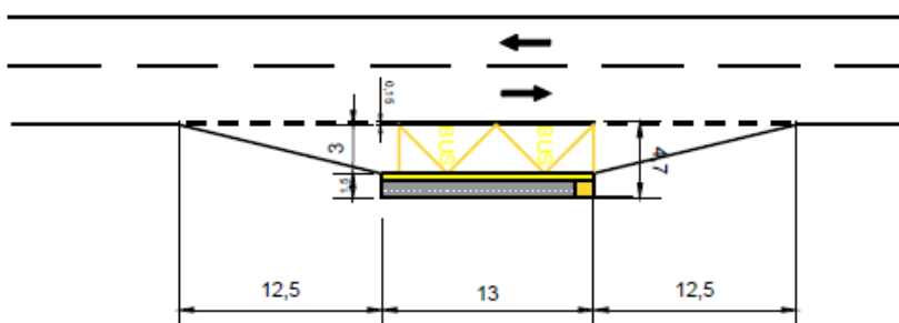
Figura 8.8: Esquema de parada con apartadero para cuando se dispone de un ancho de entre 4 y 4,95 metros ( 4 \leq A < 4,95 m). Los tramos de aceleración y deceleración de la figura se han dimensionado considerando una carretera interurbana con una velocidad de proyecto o de señalización de 40 km/h
