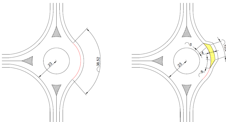
Figura 7.39: Parada urbana con apartadero en calzada anular de la rotonda
