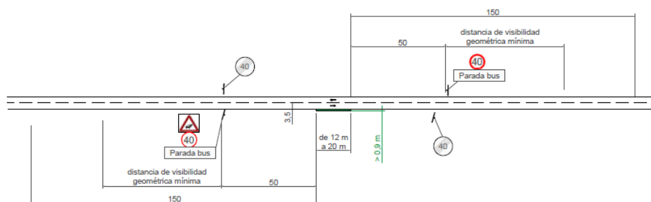
Parada interurbana sin apartadero a 40 km/h, adelantamiento permitido
