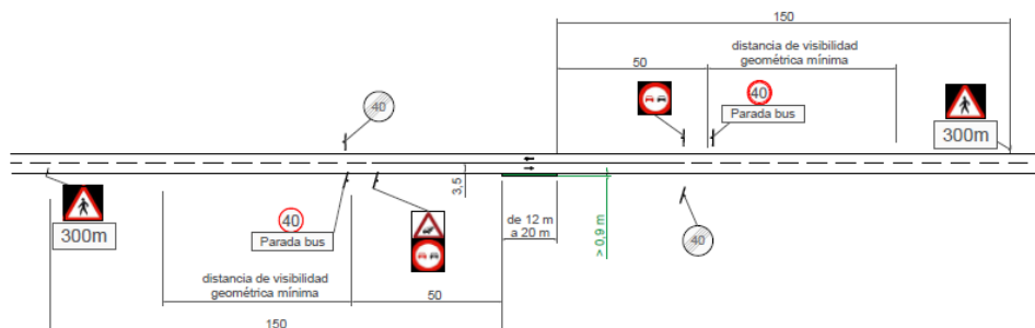
Figura 8.20: Parada interurbana sin apartadero a 40 km/h
