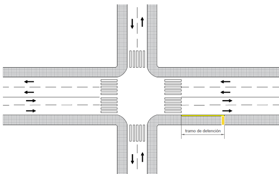
Figura 7.22: Ubicación recomendada de una parada de autobús después de una intersección con paso de peatones en calle de doble sentido y dos carriles por sentido
