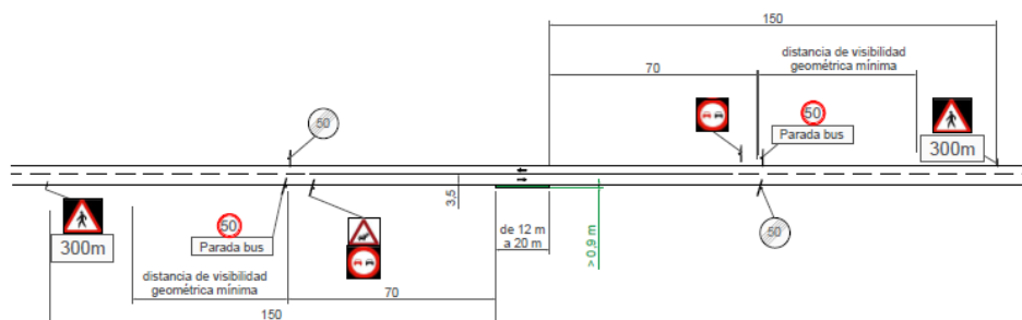
Figura 8.21: Parada interurbana sin apartadero a 50 km/h
