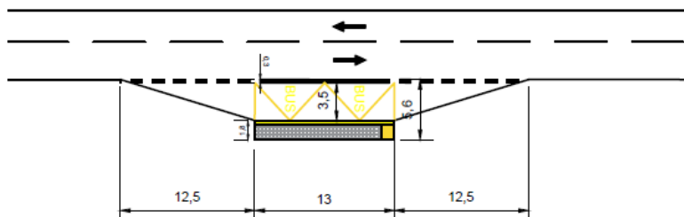
Figura 8.6: Esquema de parada con apartadero para cuando se dispone de un ancho de entre 5,45 y 5,8 metros ( 5,45 \leq A < 5,8 m). Los tramos de aceleración y deceleración de la figura se han dimensionado considerando una carretera interurbana con una velocidad de proyecto o de señalización de 40 km/h
