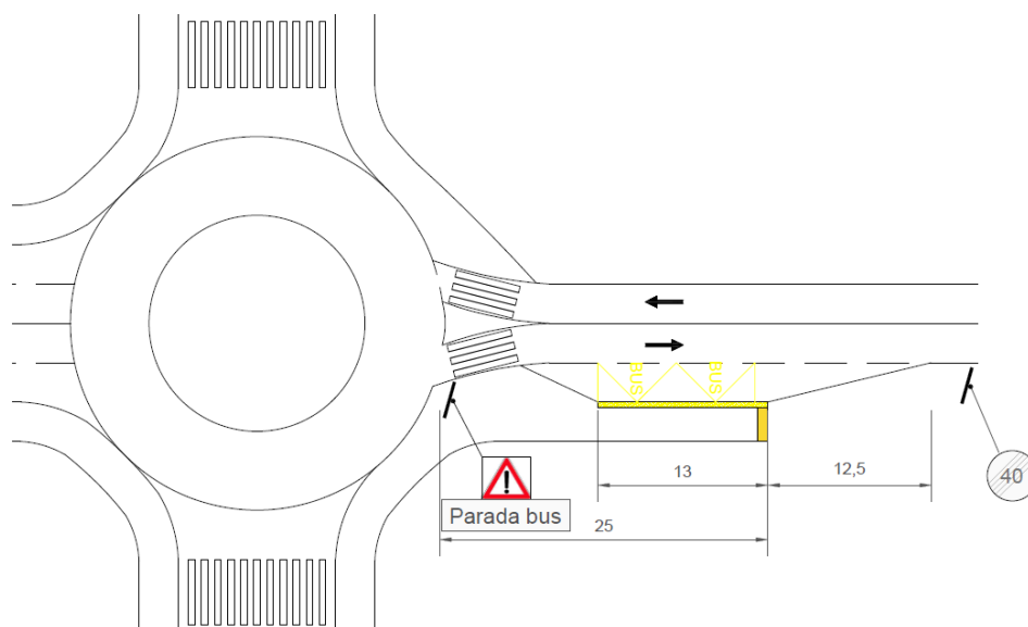
Figura 8.17: Parada interurbana con apartadero después de rotonda
