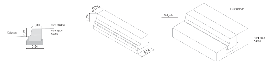
Figura 5.1: Detalle bordillo tipo Kassel
