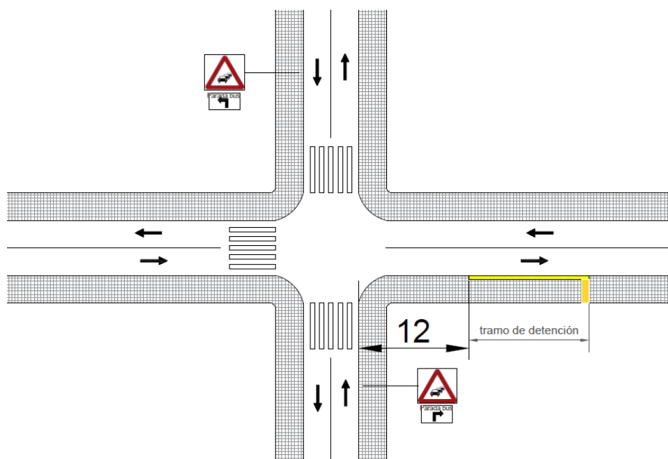
Figura 7.16: Aviso de peligro antes de intersección por parada sin apartadero después de intersección
