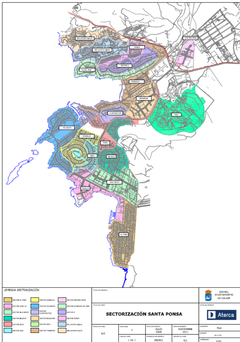
Plano zonas de distribución
