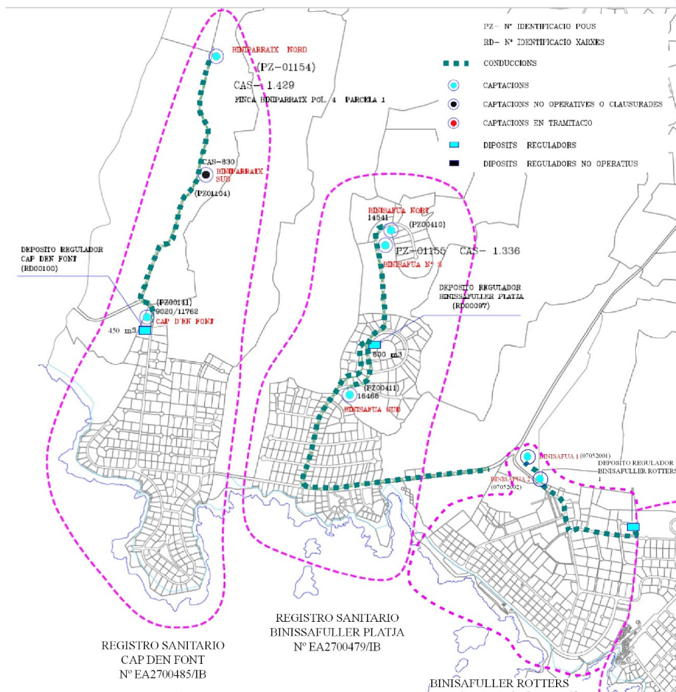
Figura 2. Sistema general d'abastament de les urbanitzacions de cap d'en Font, Binissafüller Platja i Roters. Situació de les captacions, dipòsits i conduccions en alta (Aigües Sant Lluís SL i IDE Menorca).
