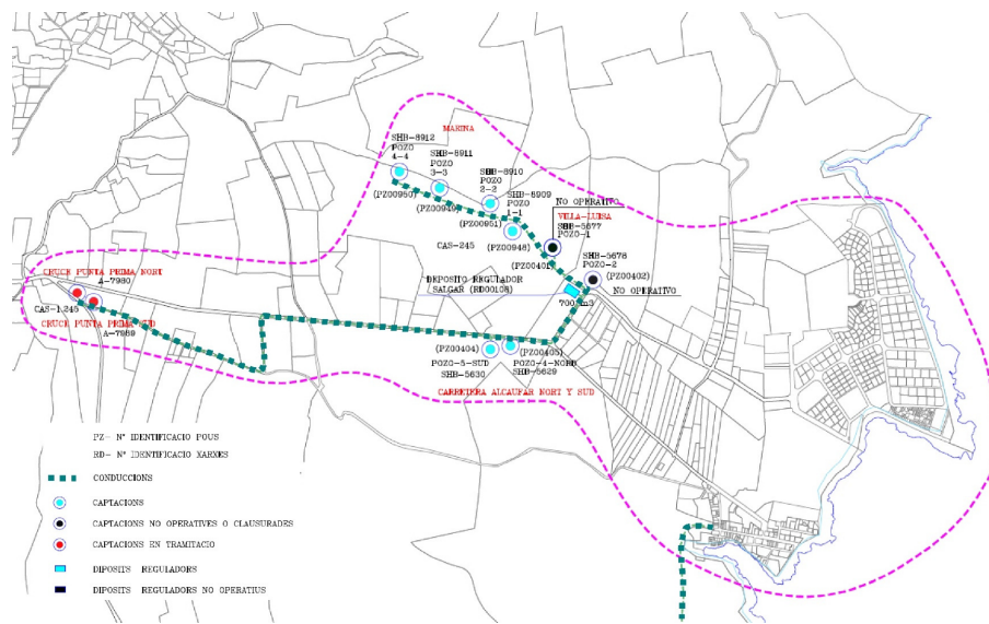
Figura 4. Sistema general d'abastament de les urbanitzacions s'Algar – Alcaufar. Situació de les captacions, dipòsits i conduccions en alta (Aigües Sant Lluís SL).
