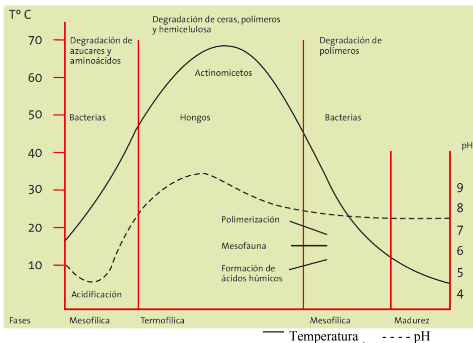
Gràfic 2: Etapes del procés de compostatge. Font: Laos, 2003; Jose M a Álvarez de la Puente
