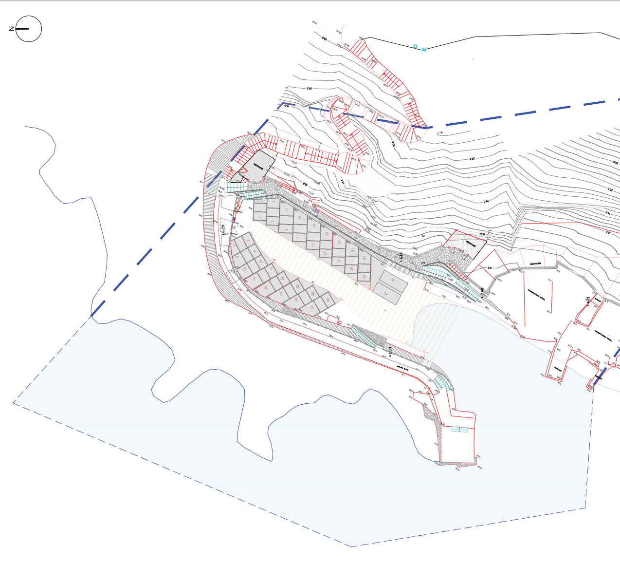
PLANTA GENERAL DEL PUERTO DE BANYALBUFAR. E:1/750
