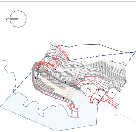
PLANTA GENERAL DEL PUERTO DE BANYALBUFAR. E:1/750
