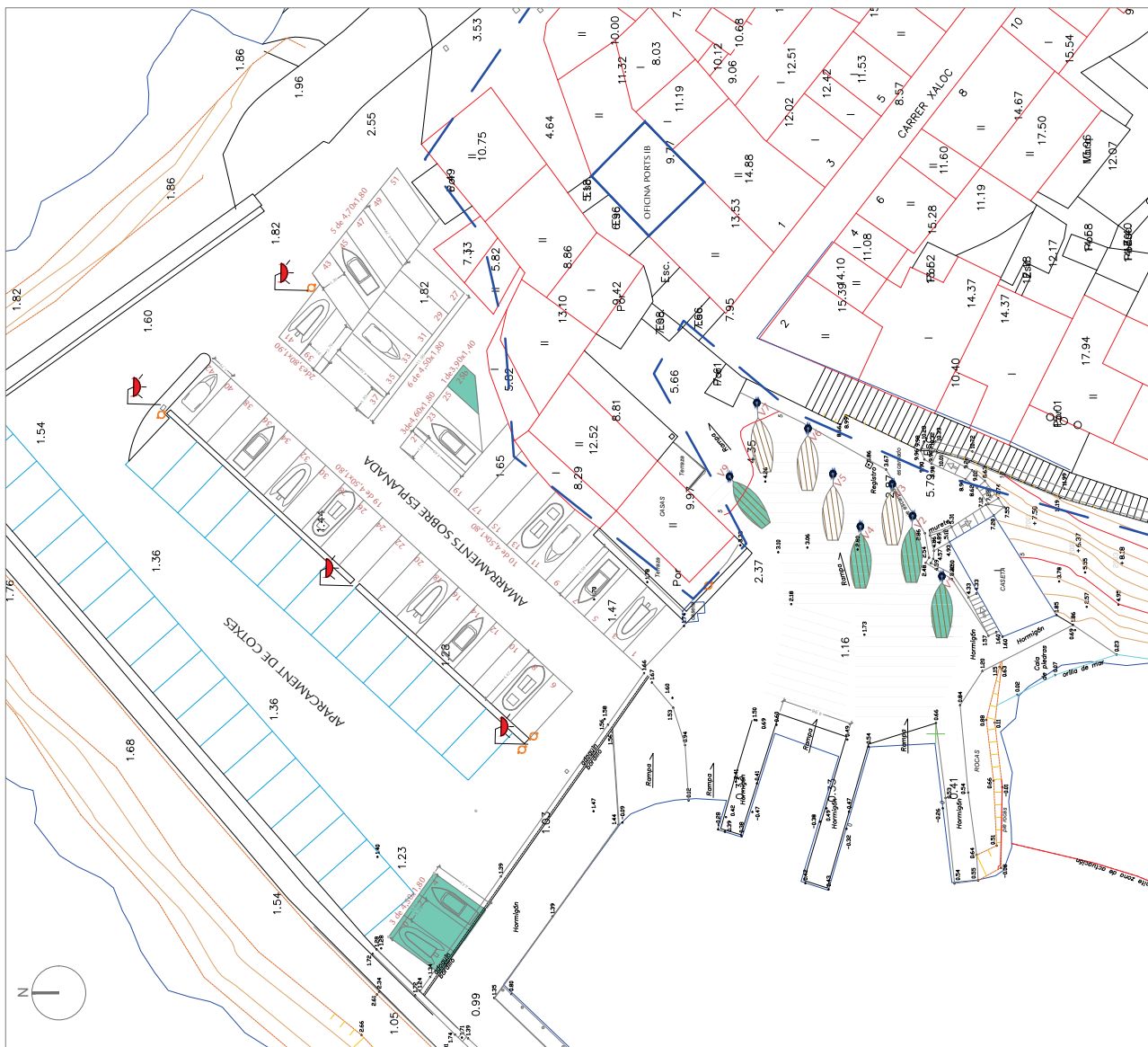
PLANTA GENERAL DEL PUERTO DE VALDEMOSA. E:1/1000
