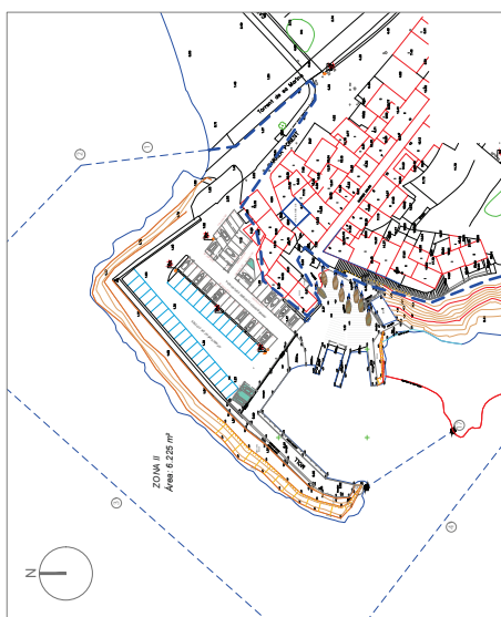
PLANTA GENERAL DEL PUERTO DE VALDEMOSA. E:1/1000
