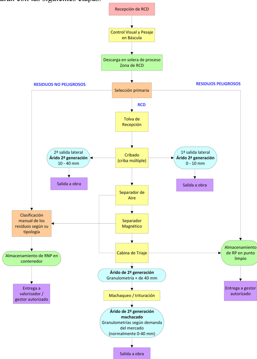
Gráfico 4: Etapas del proceso de valorización de RCD's. Fuente: GEPRECON
