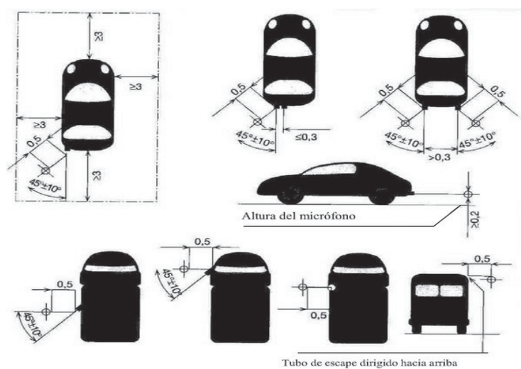
Figura 2. Posició de l'instrument de medició en vehicles automòbils
