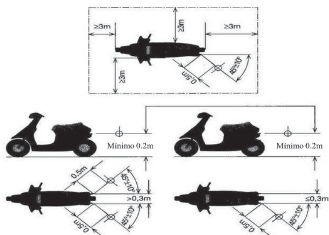
Figura 1. Posició de l'instrument de medició en ciclomotors, motocicletes i quadricicles.
