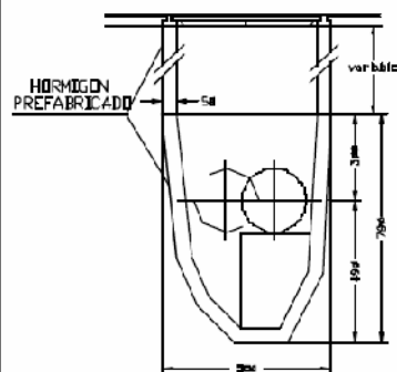
VISTA CONJUNTO ( SECCION A - A' )
