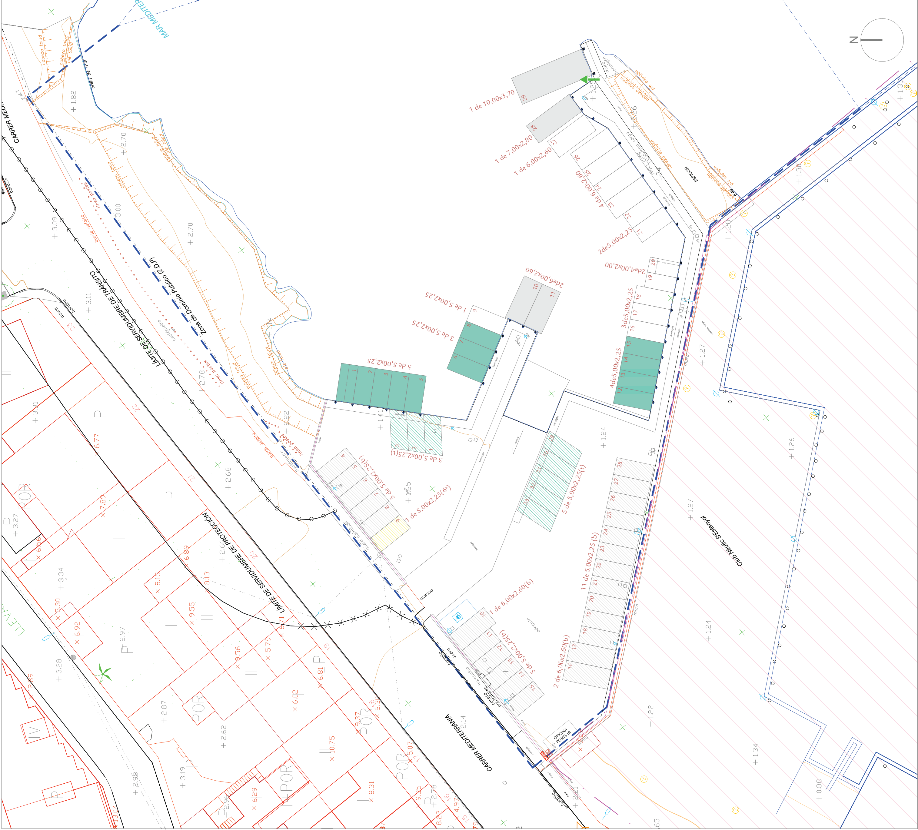
PLANTA GENERAL DEL PUERTO DE S'ESTANYOL E:1/2500
