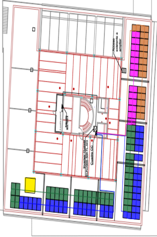
PLANTA CUBIERTA
