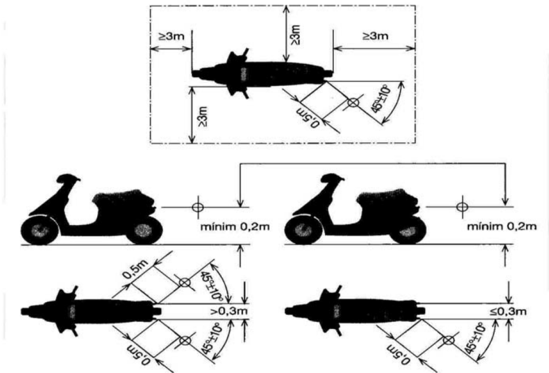
Figura 1. Posición del instrumento de medición a ciclomotores, motocicletas y cuadriciclos
